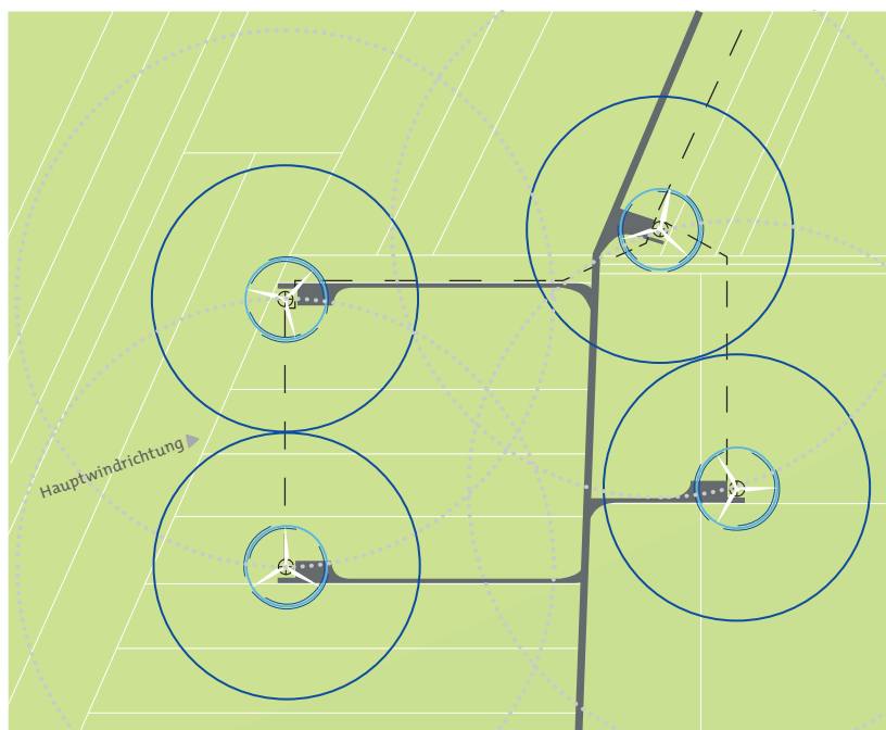
Standortplanung für einen Windpark
